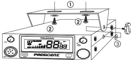
СХЕМА УСТАНОВКИ
